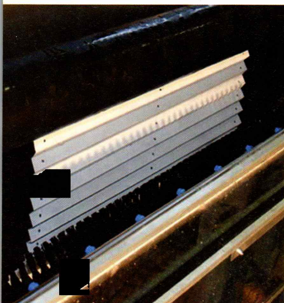
Plisseevorhang wird durch Bürstenwalzen gereinigt. Vorhang wird in TFR 2200 eingelegt. Spezialbürsten sorgen für optimale Tiefenreinigung.
